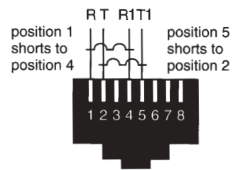
USOC RJ48X
