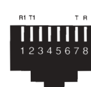
USOC RJ48S
