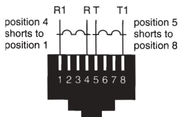
USOC RJ31X
