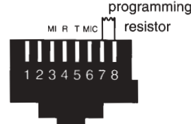
USOC RJ45S
